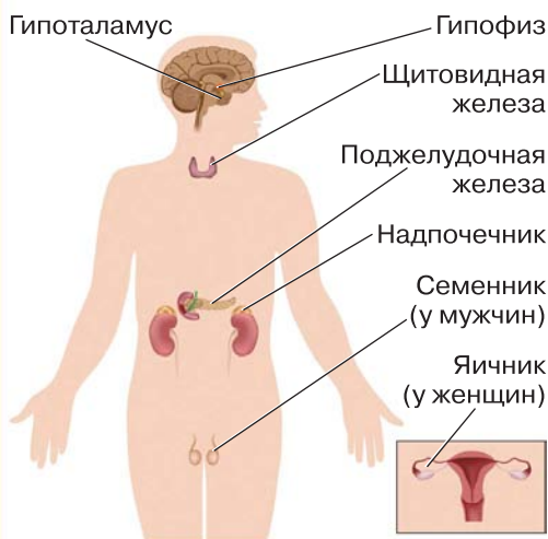
Рис. 59. Железы внутренней секреции
