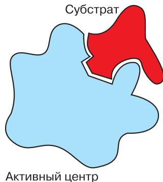
Рис. 54. Схема механизма работы фермента
